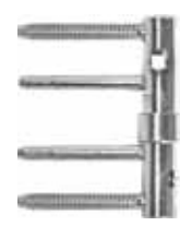
zawias z funkcją domykającą (ościeżnica drewniana stała lub regulowana jednostronnie) 66/81,18
